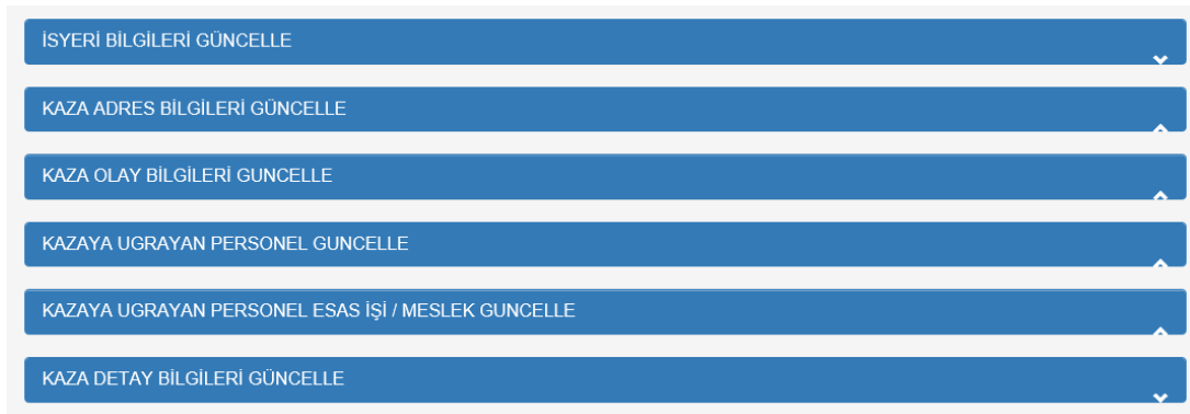
Şekil 27- Güncelleme ekranı
